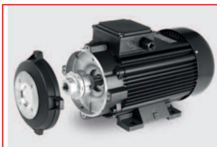
Accoppiamento motore pompa con giunto elastico
