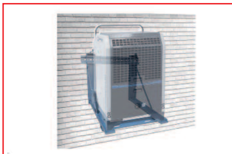
Foto 2 - Kit staffe a muro.
